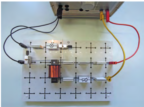
Abb. 16: Lichtsensor LDR
